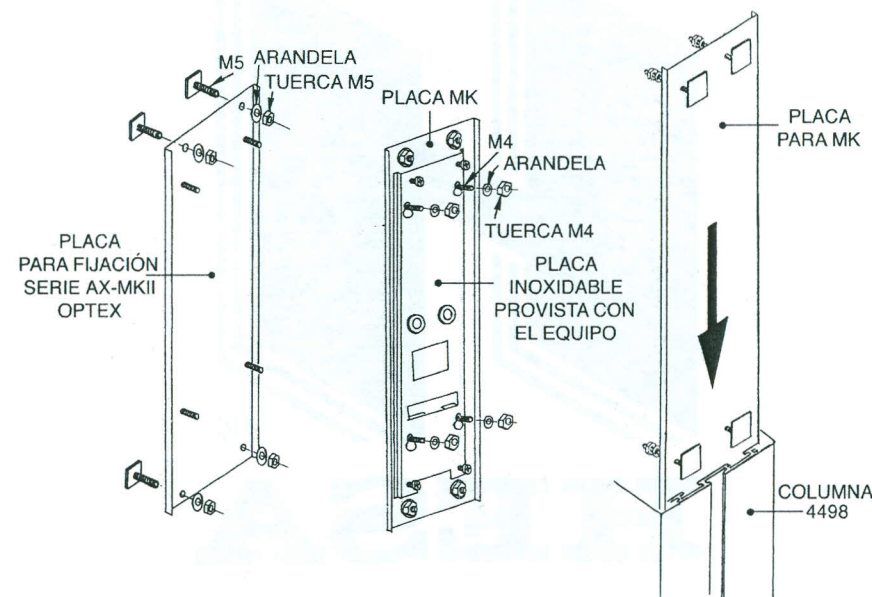
Esquema de fijación placa MK
